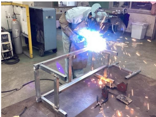
パイプ溶接
